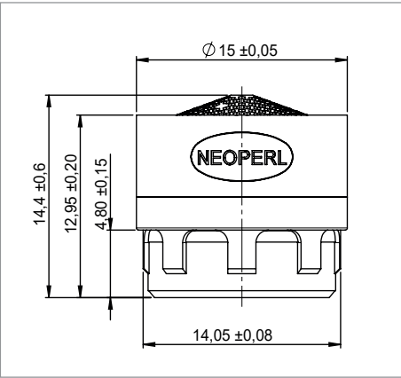
PERLATOR® HC PCA® TT insert
