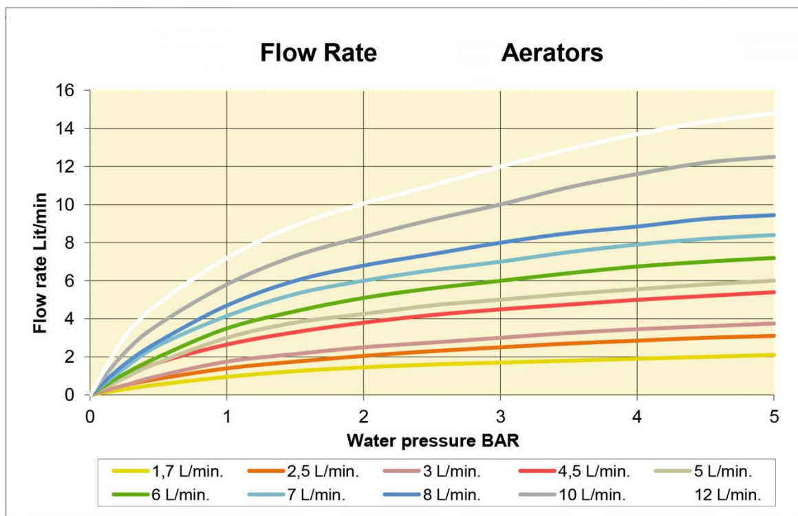
Grafico 1 – Portate d'acqua disponibili
