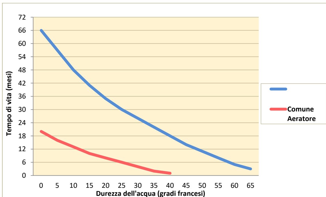
Grafico 2 – Dimostrazione della durata di funzionamento in base alla durezza dell'acqua, espressa in gradi francesi, rispetto ai comuni aeratori in commercio
