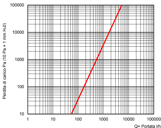
Diagramma perdite di carico
