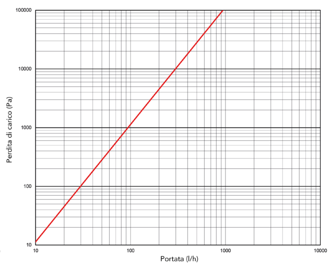
Caduta di pressione flusso in by-pass:
