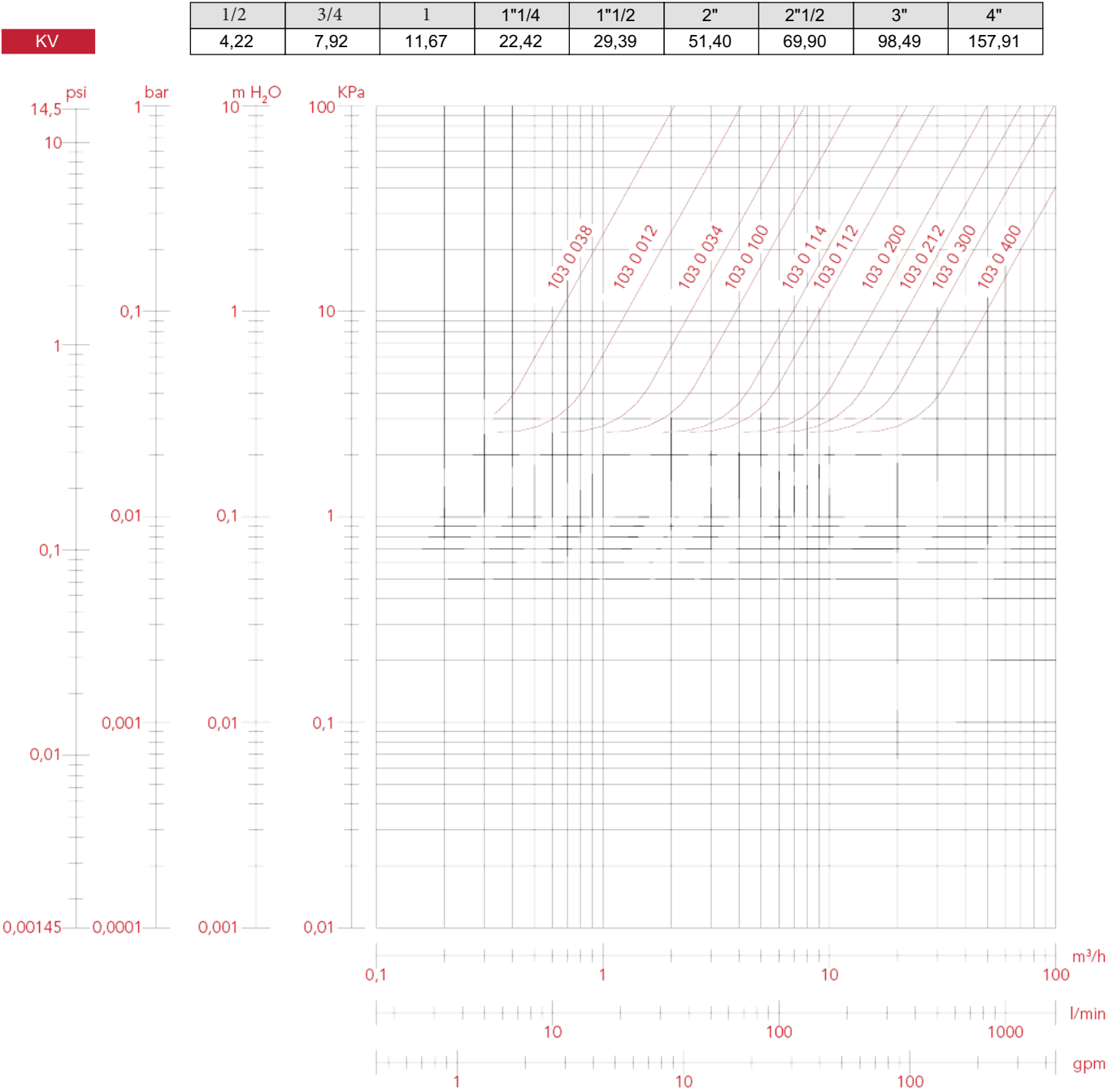
DIAGRAMMA PERDITE DI CARICO (Con acqua)
