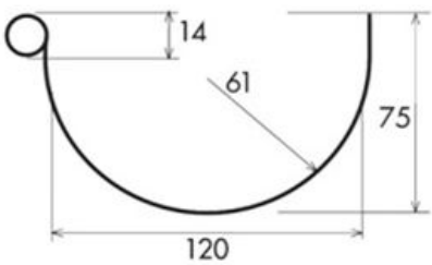
Sezione 364-TGRN
